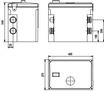
2. ábra Körvonalrajz
